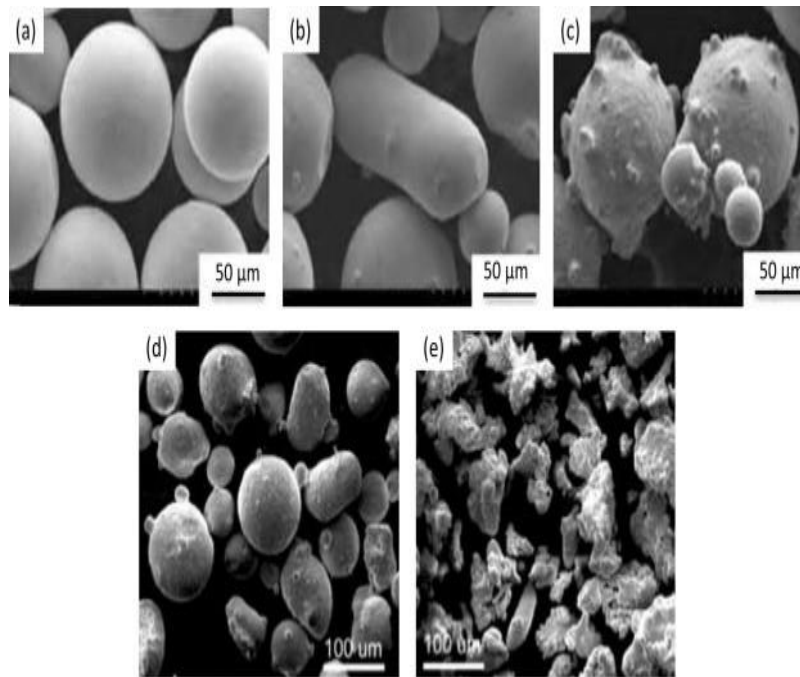
Fig. 2. Imagen de los polvos de aleación fabricados mediante el proceso (a) PREP (b) RA y (c) GA. Comparación de la forma de los polvos fabricados mediante el proceso (d) GA y (e) WA (Debroy et al., 2018)
