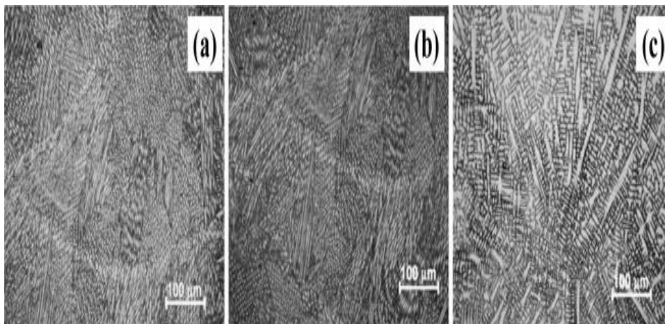
Fig.3. Microestructuras solidificadas con escalas dependientes de la altura de capa. (a) Capa inferior, (b) media y (c) superior para una estructura de 9 capas de acero inoxidable austenítico 316L de DED-L (Manvatkar et al., 2011)
