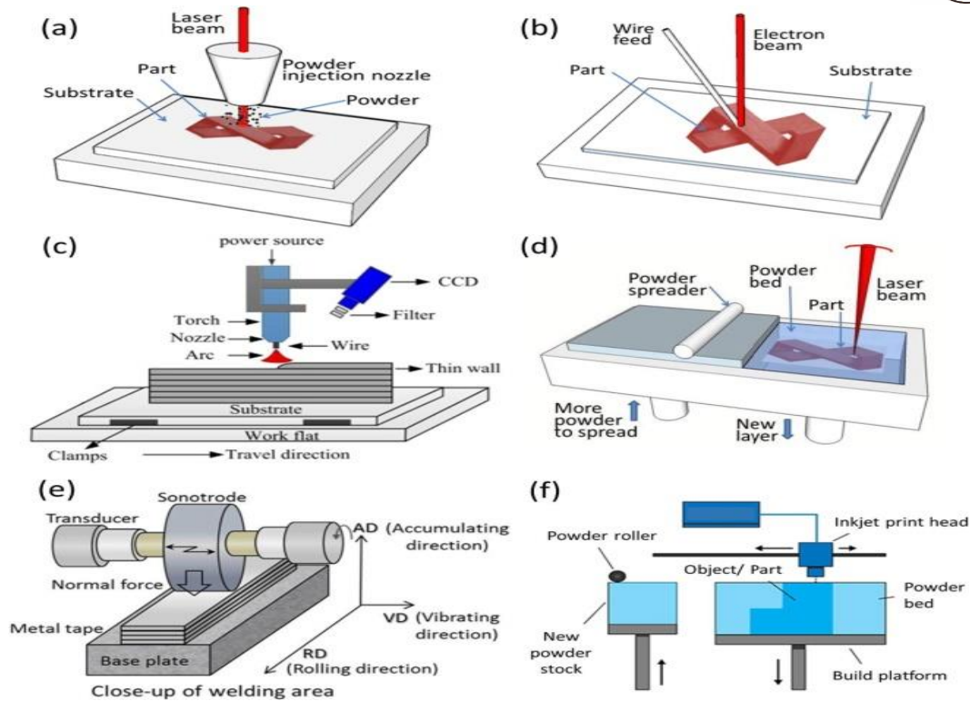
Fig.1. Diagrama esquemático de (a) DED-L (b) DED-EB (c) DED-GMA (d) PBF-L (e) proceso de fabricación aditiva ultrasónica (UAM) y (f) proceso de chorro de aglutinante (Debroy et al., 2018)
