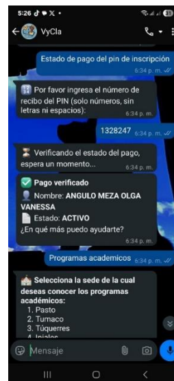
Fig. 6. Interacción de un usuario con el sistema.
