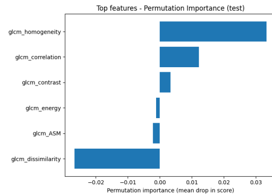
Fig. 6. Importancia de la permutación.
