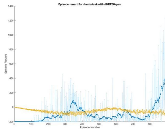
Fig. 7. Diagrama de recompensa por episodio (Recompensa por episodio en azul y Valor del Crítico en amarillo)
