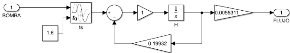
Fig. 5. Bloque de diagrama del modelo matemático
