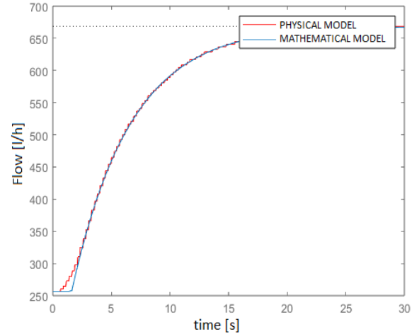
Fig. 4. Modelo físico vs modelo matemático
