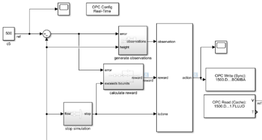
Fig. 8. Conexión de bloques por OPC
