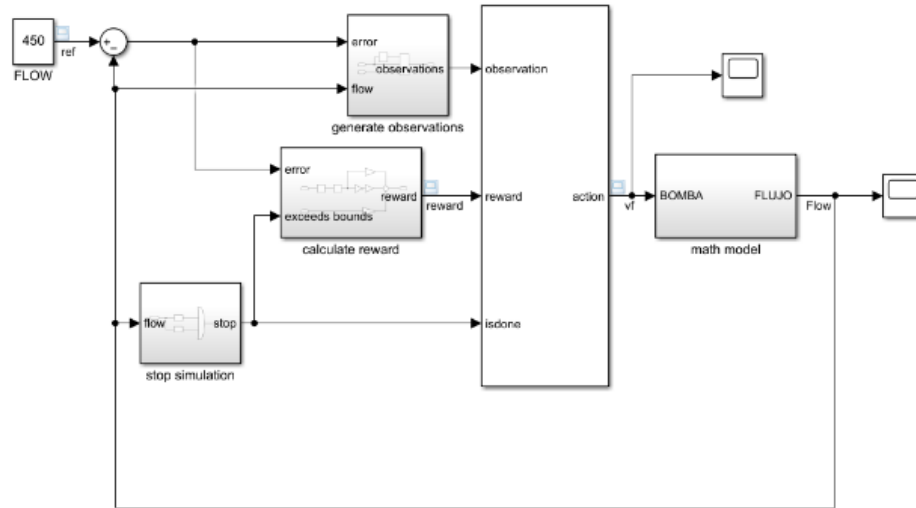
Fig. 6. Diagrama de bloques del entorno de aprendizaje
