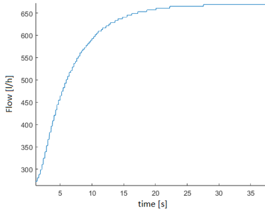
Fig. 3. Diagrama de curva de proceso
