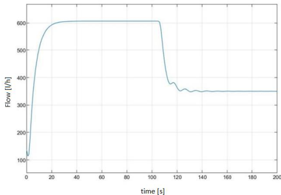
Fig. 9. Respuesta de la planta al sistema de control propuesto con dos valores de referencia
