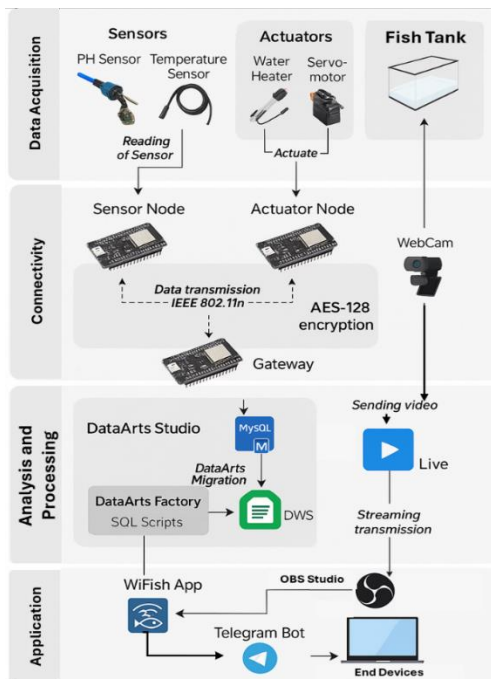
Fig. 1. Arquitectura del sistema. Fuente: elaboración propia.
