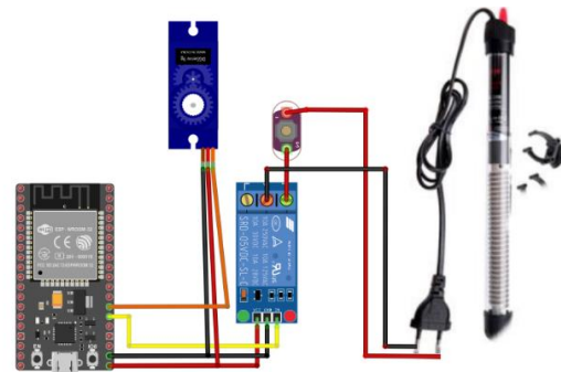
Fig. 4. Diagrama de conexión nodo actuador. Fuente: elaboración propia.
