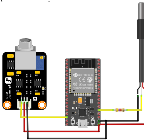
Fig. 3. Diagrama de conexión nodo sensor. Fuente: elaboración propia.
