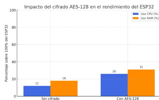
Fig. 13 Impacto del cifrado AES-128 Fuente: elaboración propia
