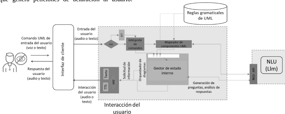
Fig. 2. Diagrama a bloques con tres zonas: (i) Entrada accesible —usuario dicta o escribe un comando UML; (ii) Procesamiento semántico —comando pasa por intérprete, mapeo UML y consulta a un LLM validado con reglas UML; (iii) Generación/gestión del modelo —estado interno persistido y respuestas en audio/texto devueltas al usuario.
