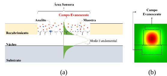
Fig. 3. Biosensores de Onda Evanescente: (a) Principio de Funcionamiento (b) Propagación Modal Fuente: elaboración propia
