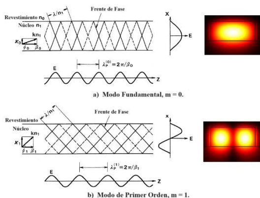
Fig. 2. Formación de los Modos de Propagación. (a) Modo Fundamental (b) Modo de Primer Orden Fuente: adaptado de [19]
