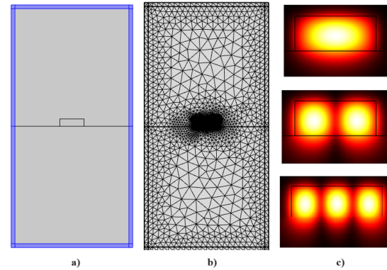
Fig. 5. Método FEM para análisis de guías de onda: (a) Geometría (b) Mallado (c) Propagación Modal
