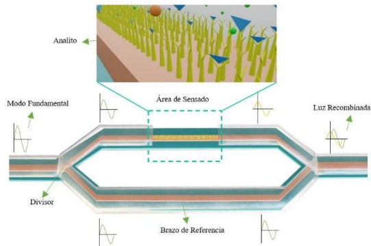
Fig. 4. Biosensor de Onda Evanescente mediante transductor MZI
