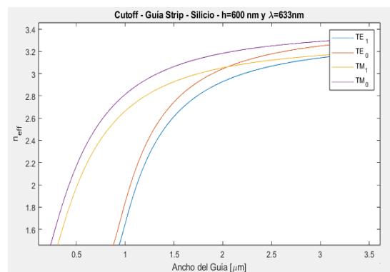
Fig. 6. Curvas de dispersión de la guía de onda Strip con núcleo de Silicio
