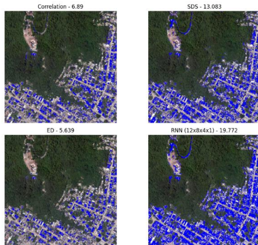
Fig. 12. Despliegue de los 4 métodos sobre la imagen multispectral de 4 bandas. Fuente: elaboración propia.
