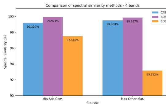
Fig. 7. Comparación de métodos de similitud espectral con píxeles de muestra de 4 bandas.
