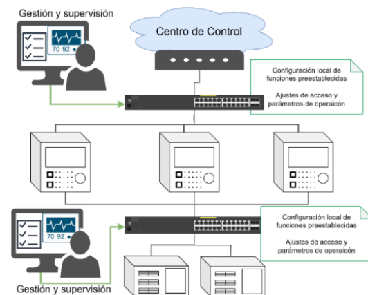
Fig. 2. Arquitectura básica para una subestación digital, compuesta por los niveles de proceso, protección y control, y el nivel de supervisión. Fuente: elaboración propia.
