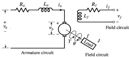
Fig. 2. Motor Brushless. Fuente: elaboración propia de [9].
