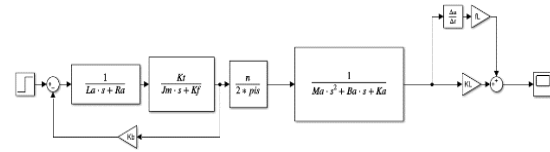
Fig. 3. Diagrama de Bloques Modelo SEA completo. Fuente: Elaboración Propia.
