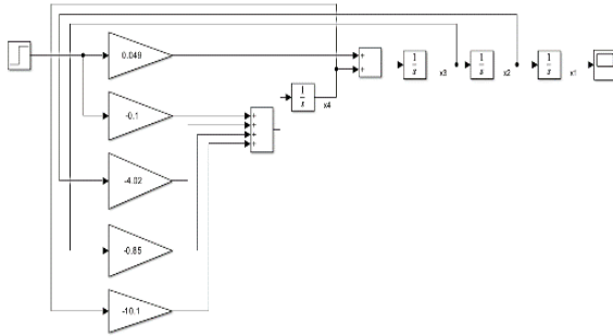
Fig. 6. Modelo SEA por representación de espacio de estados. Fuente: Elaboración Propia.
