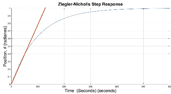
Fig. 7. Curva de reacción PID SEA. Fuente: Elaboración Propia.
