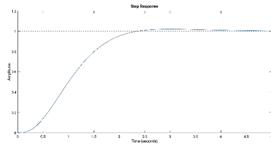
Fig. 9. Respuesta Control RVE por ubicación de polos. Fuente: Elaboración Propia.
