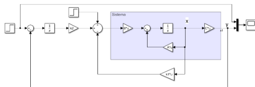
Fig. 12. Observador de Estado. Fuente: Elaboración Propia.
