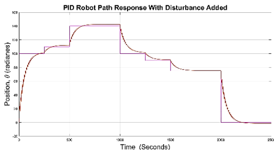
Fig. 11. Respuesta del control PID con perturbación. Fuente: Elaboración Propia.
