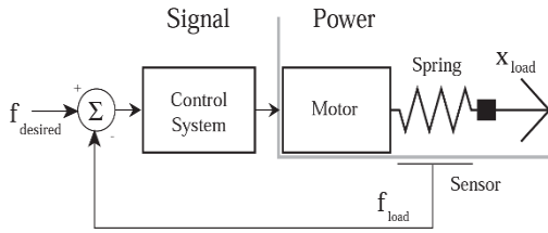
Fig. 1. Componentes SEA. Fuente: tomado de la referencia [7].
