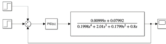
Fig. 10. PID con perturbación. Fuente: Elaboración Propia.
