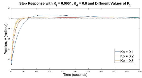
Fig. 8. Sintonización PID SEA. Fuente: Elaboración Propia.
