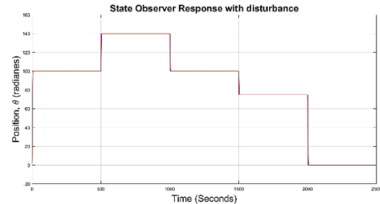
Fig. 13. Respuesta SEA Observador de Estado Fuente: Elaboración Propia.
