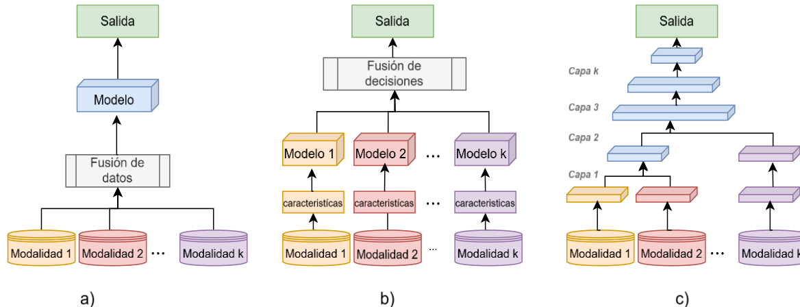
Fig. 1. En problemas multimodales, hay tres tipos de fusión: a) Fusión temprana, que combina las modalidades al inicio en un solo vector; b) Fusión intermedia, que aprende representaciones de estas modalidades antes de fusionarlas para que el modelo pueda aprender de ellas en conjunto; y c) Fusión tardía, que combina las predicciones hechas por cada modelo para sus modalidades correspondientes.
