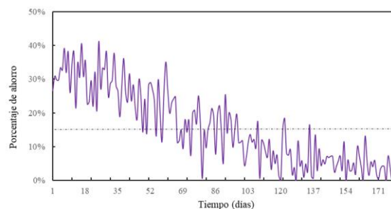
Fig. 4. Comportamiento en % de ahorro energético del sistema BFT_AUT. Fuente: Elaboración propia.
