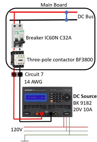
Fig. 2. Ensayo voltímetro-amperímetro (Caída de potencial). Fuente: elaboración propia.
