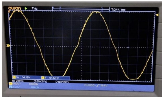
Fig. 6. Voltaje de salida del módulo de potencia tipo Puente completo SPM-FB operando como un inversor. Fuente: elaboración propia.
