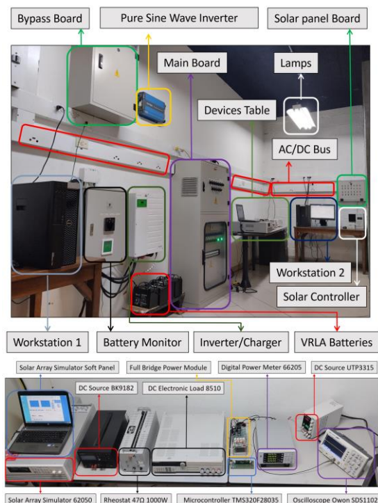
Fig. 1. Laboratorio Flexible con múltiples componentes. Fuente: elaboración propia.
