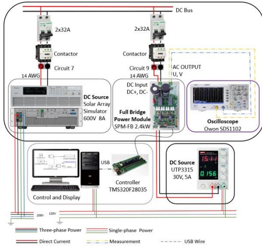
Fig. 3. Setup experimental para probar el convertidor en la operación en vacío. Fuente: elaboración propia.
