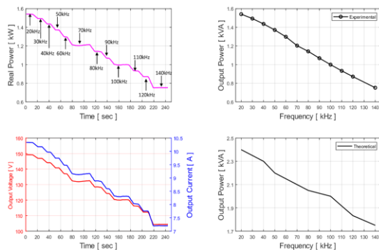
Fig. 7. Potencia vs frecuencia de conmutación durante la operación con carga del módulo de potencia puente completo. Fuente: elaboración propia.
