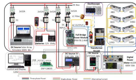
Fig. 13. Microrred de laboratorio emulando la microrred real de Isla Fuerte. Fuente: elaboración propia.
