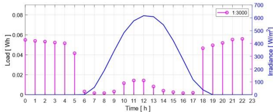
Fig. 11. Curva escalada de demanda promedio de Isla Fuerte y curva de irradiación promedio de Julio. Fuente: elaboración propia.
