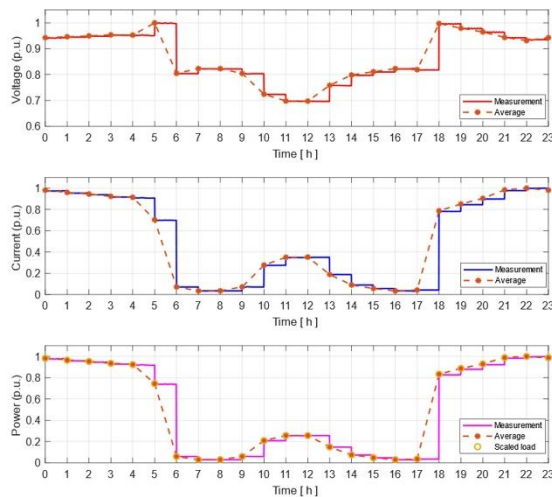
Fig. 14. Voltaje, corriente y potencia en la carga de la microrred emulada de Isla Fuerte. Fuente: elaboración propia.
