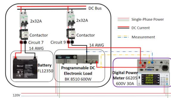
Fig. 8. Setup experimental para descargar las baterías bajo una prueba con un perfil de referencia. Fuente: elaboración propia.
