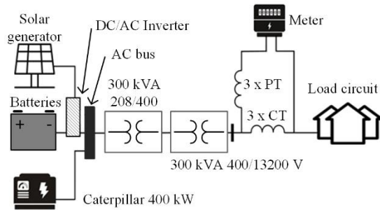
Fig. 12. Esquemático de la microrred que opera en Isla Fuerte. Fuente: elaboración propia.
