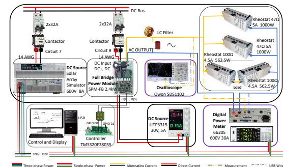
Fig. 5. Setup experimental para probar el convertidor de potencia en la operación con carga. Fuente: elaboración propia.
