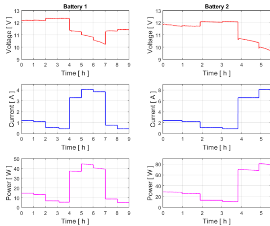
Fig. 9. Voltaje, corriente y potencia de dos baterías bajo una prueba con un perfil de referencia. Fuente: elaboración propia.
