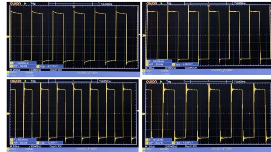
Fig. 4. Voltaje de salida del convertidor en vacío durante la variación de frecuencia. Fuente: elaboración propia.
