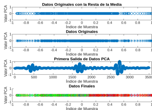
Fig. 8. Válvula Tricúspide Con Procesamiento - Análisis De Componentes Principales
