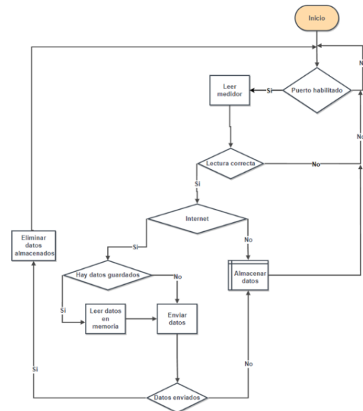
Fig. 2. Diagrama de flujo de algoritmo propuesto para la solución. Fuente: elaboración propia
