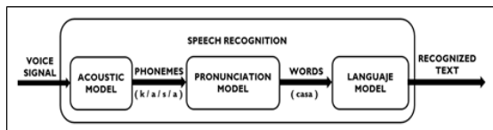
Fig. 2. Diagrama de bloques del reconocimiento de voz. Fuente: elaboración propia.
