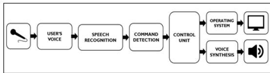
Fig. 1. Diagrama de bloques del sistema. Fuente: elaboración propia.
