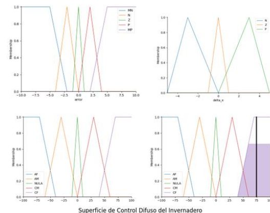
Superficie de Control Difuso del Invernadero
