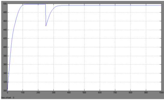
Fig. 10. Respuesta del control difuso implementado en Simulink con un step de 500 y una perturbación de 50 a las 250 mseg.
