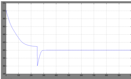
Fig. 11. Respuesta del control difuso implementado en simulink con un step de 400 y una perturbación de 50 a los 250 mseg.
