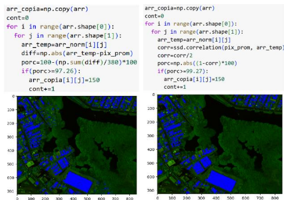
Fig. 7. Detección de asbesto sobre la imagen hiperespectral de referencia mediante los métodos de similitud diferencial y correlación.
