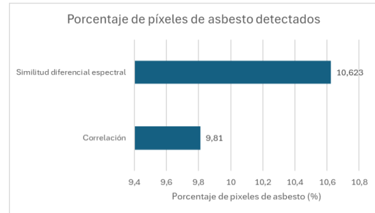
Fig. 8. Porcentaje de píxeles de asbesto detectados. Fuente: elaboración propia.
