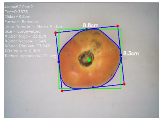
Fig. A-11. Tomate No11 procesado por el algoritmo. Fuente: Elaboración propia
