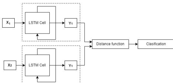
Fig. 4. Arquitectura de red Siamese-LSTM Fuente: (adaptada de [4])
