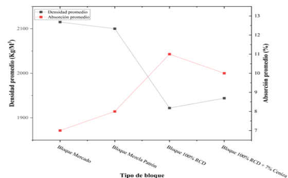
Fig. 8. Resultados de densidades y porcentajes (%) de absorción de los bloques de concreto.
