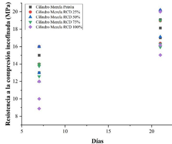
Fig. 6. Resistencia a la compresión inconfiada cilindros patrón y con adición RCD Fuente: elaboración propia.
