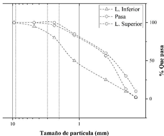
Fig. 3. Granulometría arena fina Fuente: elaboración propia.
