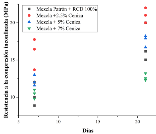
Fig. 7. Cilindros con 100% RCD + % de microperlas.
