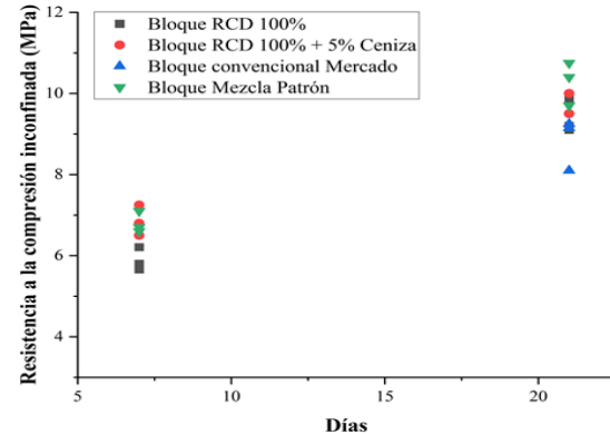
Fig. 8. Resultados compresión bloques de concreto en sus diferentes presentaciones.
