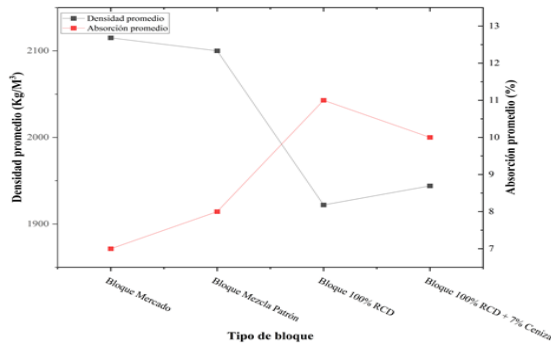
Fig. 8. Resultados de densidades y porcentajes (%) de absorción de los bloques de concreto.
