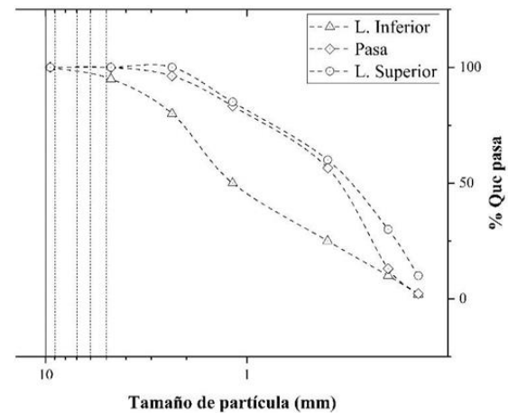
Fig. 4. Granulometría arena gruesa Fuente: elaboración propia.
