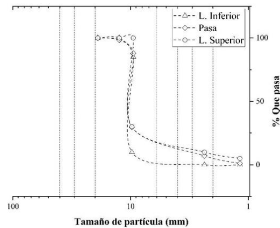
Fig. 5. Granulometría RCD. Fuente: elaboración propia.
