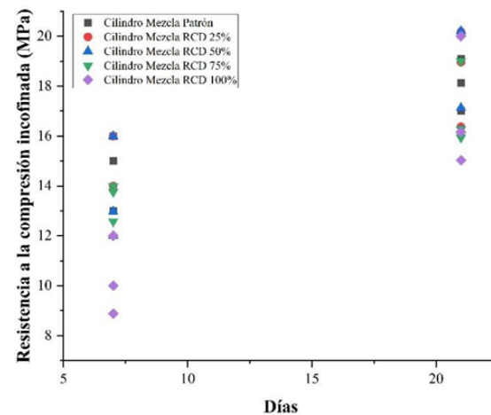
Fig. 6. Resistencia a la compresión inconfiada cilindros patrón y con adición RCD
