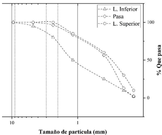
Fig. 3. Granulometría arena fina Fuente: elaboración propia.
