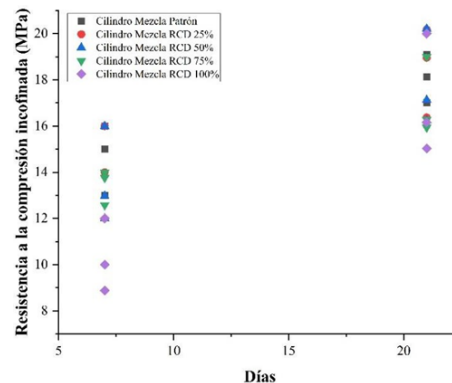
Fig. 6. Resistencia a la compresión inconfiada cilindros patrón y con adición RCD Fuente: elaboración propia.
