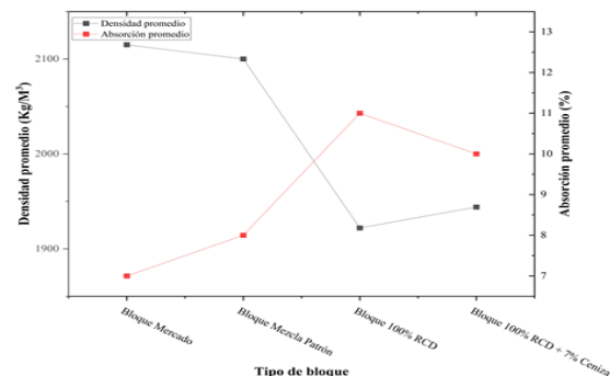
Fig. 9. Resultados de densidades y porcentajes (%) de absorción de los bloques de concreto.
