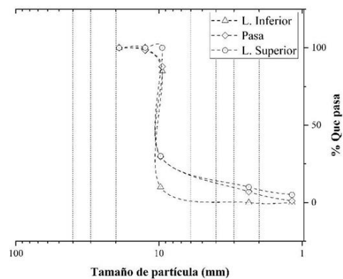
Fig. 5. Granulometría RCD. Fuente: elaboración propia.
