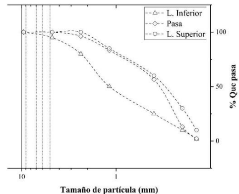
Fig. 4. Granulometría arena gruesa Fuente: elaboración propia.
