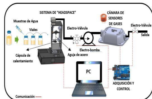
Figura 1 Esquema general de la metodología implementada. (Bacterias en agua potable a través de una nariz electrónica y un equipo de extracción de volátiles Jennifer Katherine Carrillo Gómez et al., n.d.)
