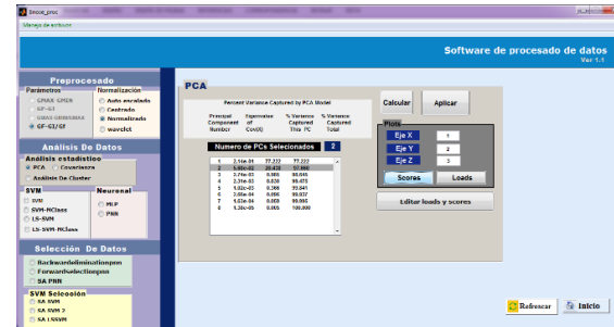
Figura 92 Análisis PCA (imagen propia)
