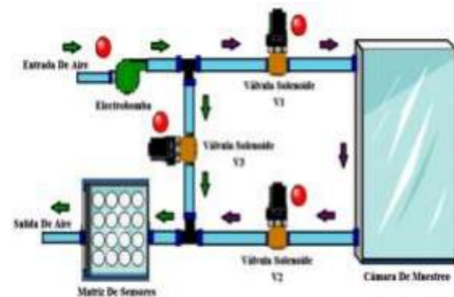
Figura 5 Nariz Electrónica E-Nose Universidad de Pamplona
