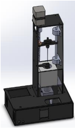
Figura 2 Diseño del headspace sampling (imagen propia)
