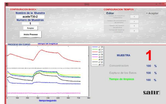
Figura 7 Respuesta de los sensores a 30°C
