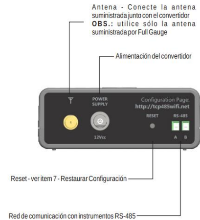
Fig. 8. Conexión RS-485 convertidor
