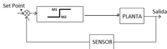
Fig. 2. Diagrama de bloques de un sistema de control ON/OFF
