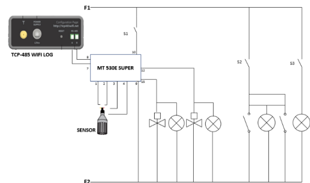
Fig. 9. Plano eléctrico
