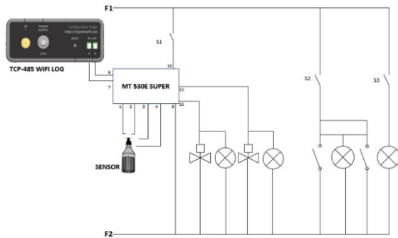
Fig. 9. Plano eléctrico
