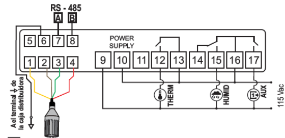
Fig. 7. Conexiones eléctricas MT530e super
