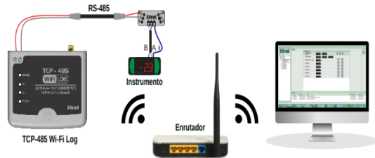
Fig. 6. Esquema de conexión controlador-convertidor- computador
