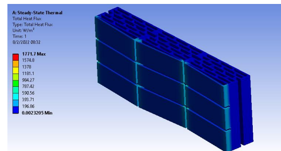
Fig. 8. Resultados de flujo de calor superficie exterior.
