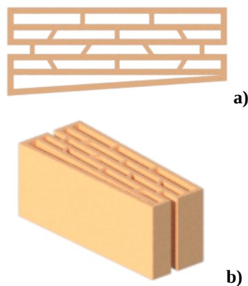
Fig. 2. Diseño Unidad Constructiva: (a) Planta (b) Isometría.
