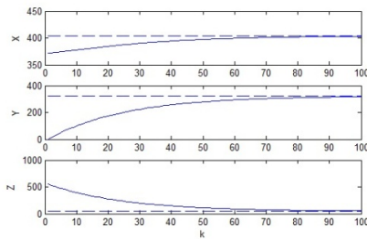
Fig. 4a. Variación del punto x,y,z del robot simulado.
