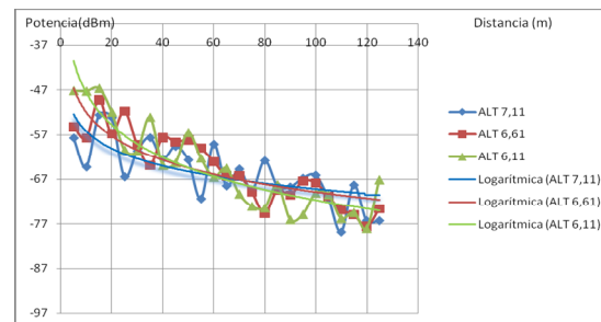
Fig. 7: Niveles de potencia ambiente sub urbano 3 (ruta 1), 100mW variación de altura 6.11, 6.61 y 7.11 metros.
