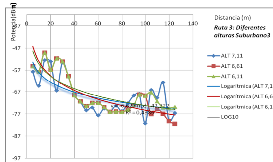
Fig. 7: Niveles de potencia ambiente sub urbano 3 (ruta 3), 100mW variación de altura 6.11, 6.61 y 7.11 metros
