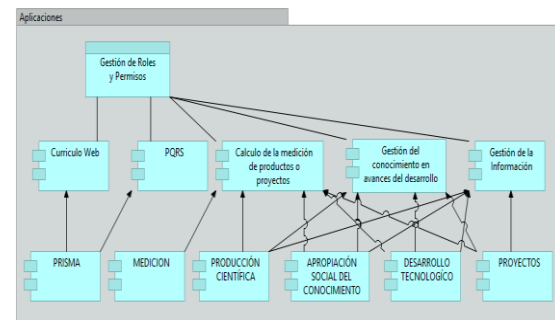
Fig. 7. TO-BE del Modelo de Funcionalidades para la Arquitectura de Aplicaciones.
