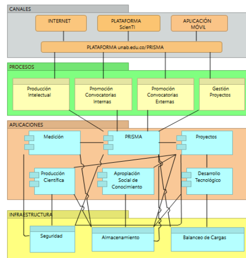
Fig. 4. Solución a Alto Nivel del Modelo Arquitectónico AE.
