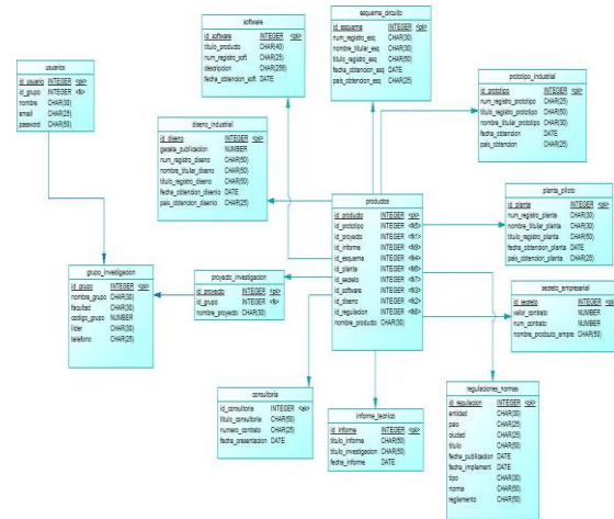
Fig. 6. Modelo Relacional TO-BE – Productos Desarrollo Tecnológico e Innovación.
