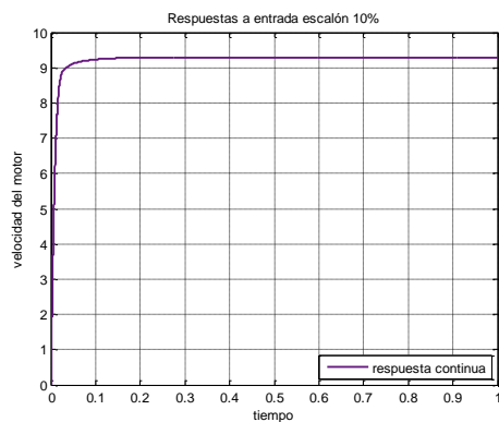
Fig. 15. Respuesta de velocidad del motor con un control PD difuso en tiempo continuo ante una entrada de 10%
