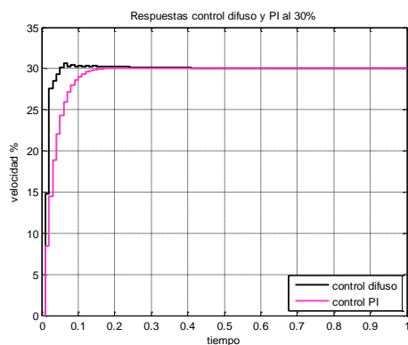
Fig. 20. Respuesta de velocidad del motor con un control PI difuso y PI clásico en tiempo discreto ante una entrada de 30%
