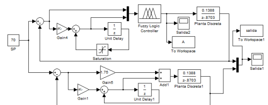
Fig. 14. Diagrama de bloques de la comparación del control PI y el control difuso en Matlab simulink®
