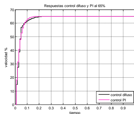
Fig. 18. Respuesta de velocidad del motor con un control PI difuso y PI clásico en tiempo discreto ante una entrada de 65%
