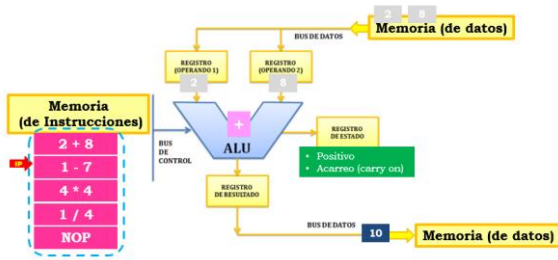
Fig. 2. Ejecución de la instrucción por parte de la ALU. Fuente: los autores
