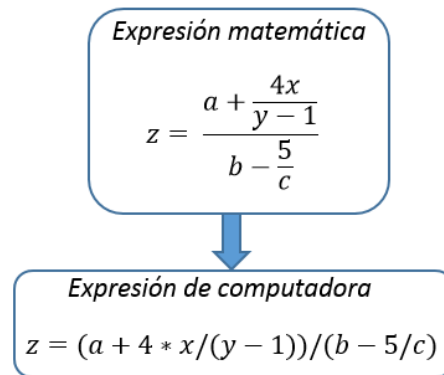
Fig. 6. Traducción de expresiones matemáticas a expresiones de computadora. Fuente: los autores.
