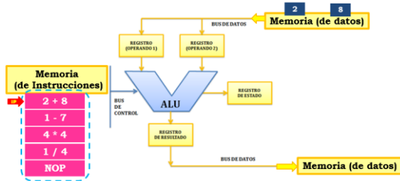
Fig. 1. Preparación de la instrucción a ser ejecutada por la ALU. Fuente: los autores
