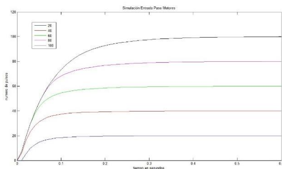
Figura 11. Gráfica de distintos valores de entradas paso ingresadas a un motor con controlador
