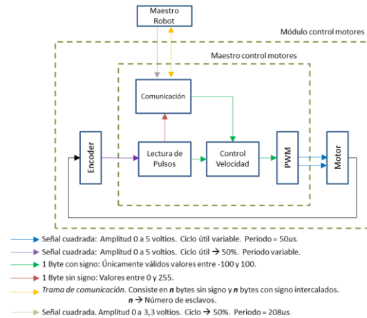
Figura 3. Módulo control de motores
