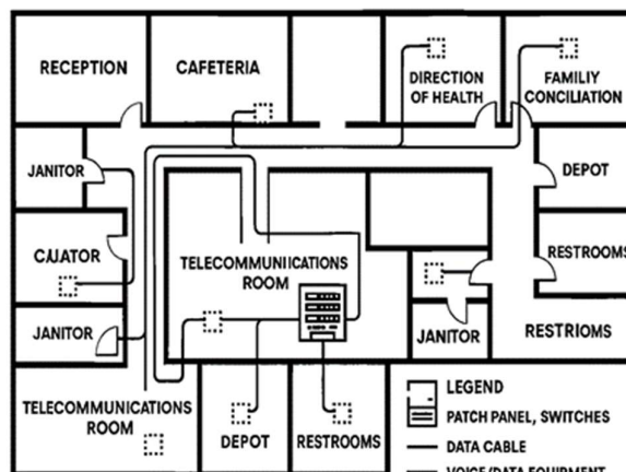
Figura 6. Distribución del proyecto. Layout Piso Uno.
