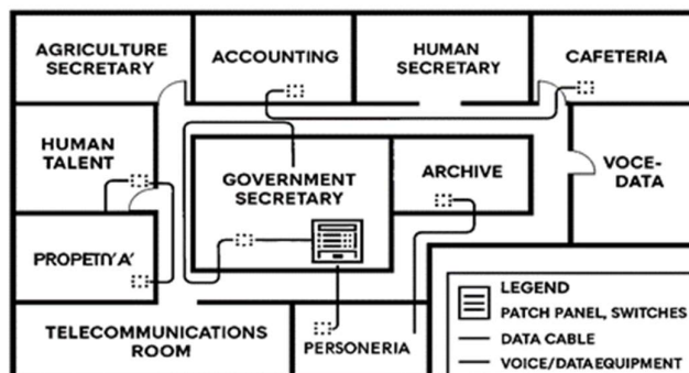
Figura 7. Distribución del proyecto. Layout Piso Dos.
