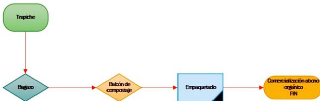
Figura 3: Estrategia de producción más limpia en el proceso de la molienda del residuo de bagazo.
