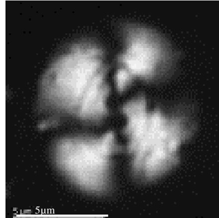
Figura 3. Muestra sección 1. Especie e: Watznaueria biporta . Lámina fotográfica en niculos cruzados. Fuente: Autores.
