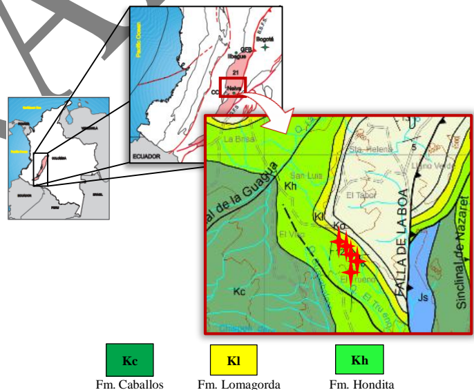
Figura 1. Localización de la zona de estudio. Fuente: Modificada de [73] y [74].
