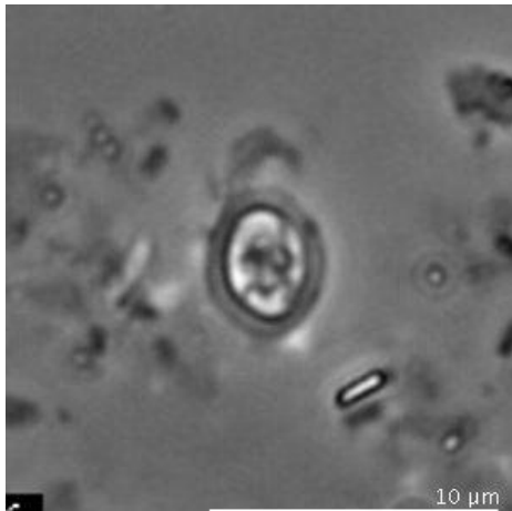
Figura 4. Muestra sección 1. Especimen de Eiffellithus spp. Lámina fotográfica en nicoles cruzados. Fuente: Autores.
