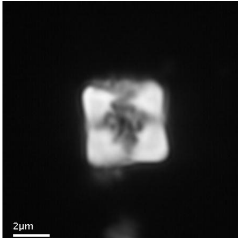
Figura 8. Muestra sección 5. Especie a: Quadrum svabnickae . Lámina fotográfica en nicoles cruzados. Fuente: Autores.
