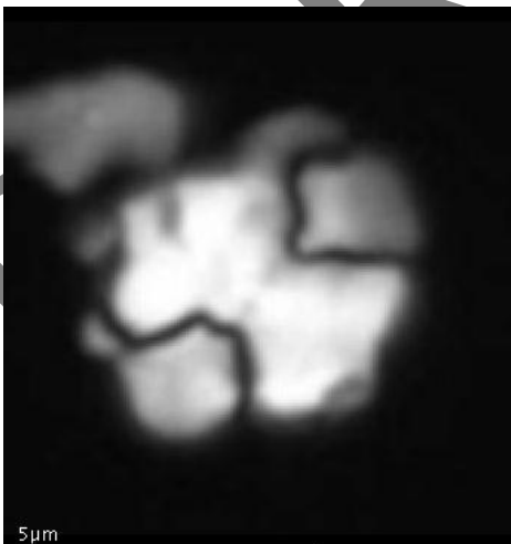
Figura 5. Muestra sección 1. Especie c: Calculites obscurus . Lámina fotográfica en nicoles cruzados. Fuente: Autores.
