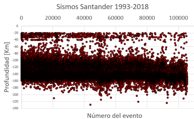
Figura 7: Distribución en profundidad de la sismicidad en el departamento de Santander para el periodo 1993-2018. Los sismos están graficados en orden cronológico. (Fuente: Autores.)
