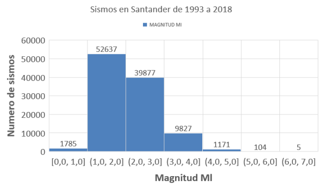
Figura 6: Histograma de la sismicidad en el departamento de Santander para el periodo 1993-2018. (Fuente: Autores.)
