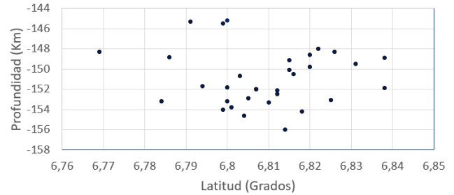
Figura 8: Distribución en latitud y profundidad de los 32 sismos para el periodo 2008 – 2018. (Fuente: Autores.)
