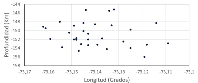
Figura 9: Distribución en longitud y profundidad de los 32 sismos para el periodo 2008 – 2018. (Fuente: Autores.)
