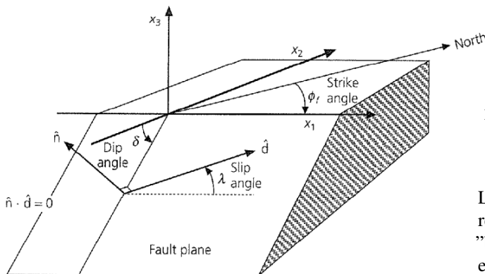
Figura 2: Parámetros y ángulos de una falla. (Imagen tomada de [12])
