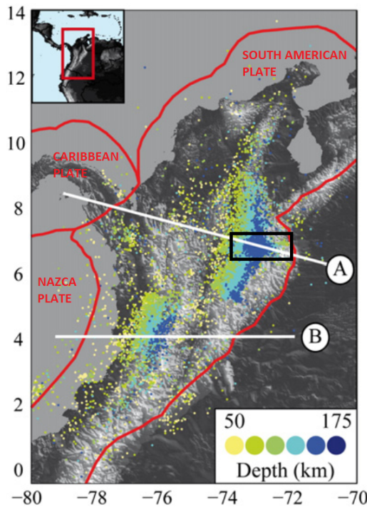
Figura 5: Sismicidad en Colombia basada en el catálogo RSNC (Red Sismológica Nacional de Colombia) codificado por colores por profundidad. La vista del mapa muestra los principales límites de las placas tectónicas. (Imagen modificada de [9])
