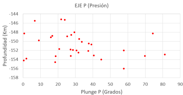
Figura 11: Representación de los ángulos de inmersión (Plunge) del eje de esfuerzos P. (Fuente: Autores.)
