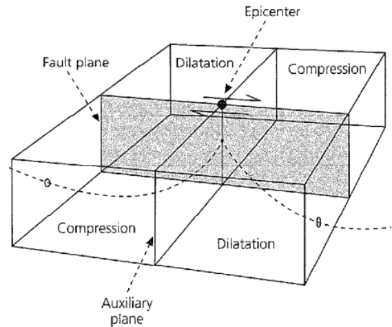
Figura 3: Planos nodales y cuadrantes para las zonas de compresión y extensión. (Imagen tomada de [12])
