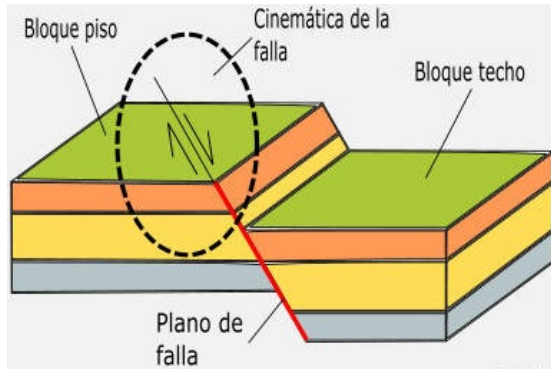
Figura 1: Elementos estructurales de una falla. (Imagen tomada de [2])
