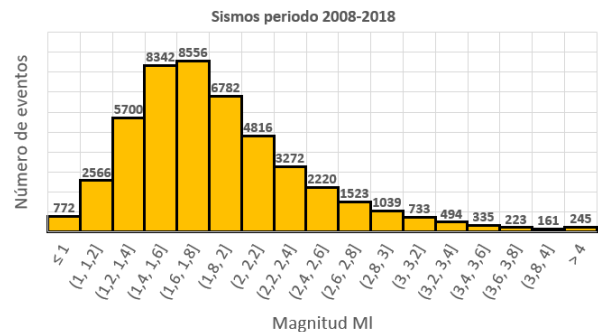
Figura 10: Histograma de la actividad sísmica para el periodo 2008 – 2018. En el rango de profundidad de 140 Km a 160 Km.
