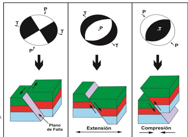
Figura 4: Balones de playa asociados al mecanismo focal de los tres tipos de fallas principales (transcurrente, normal e inversa, respectivamente). (Imagen tomada de [2])
