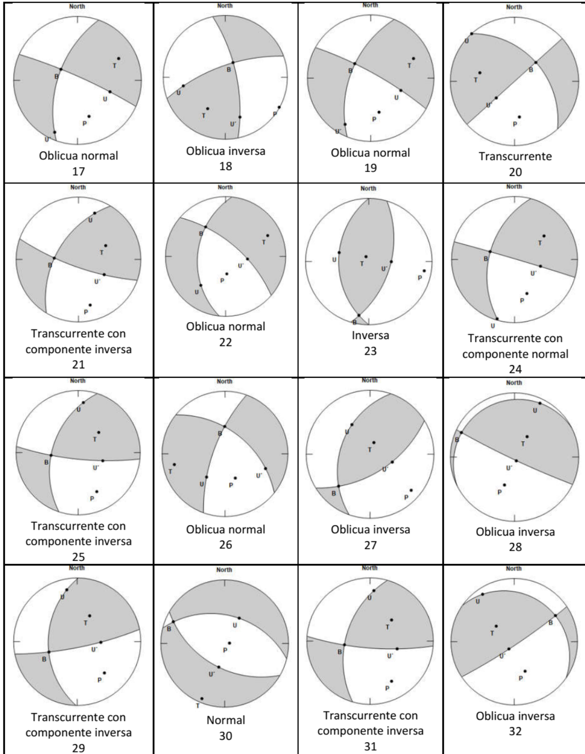
Figura 14: Gráficos de los balones de playa para los 32 sismos seleccionados. La numeración corresponde al orden de los sismos en la tabla 1, en la parte inferior se especifica el tipo de falla asociada a cada diagrama, según los parámetros de la tabla 2. (Fuente: Autores.)
