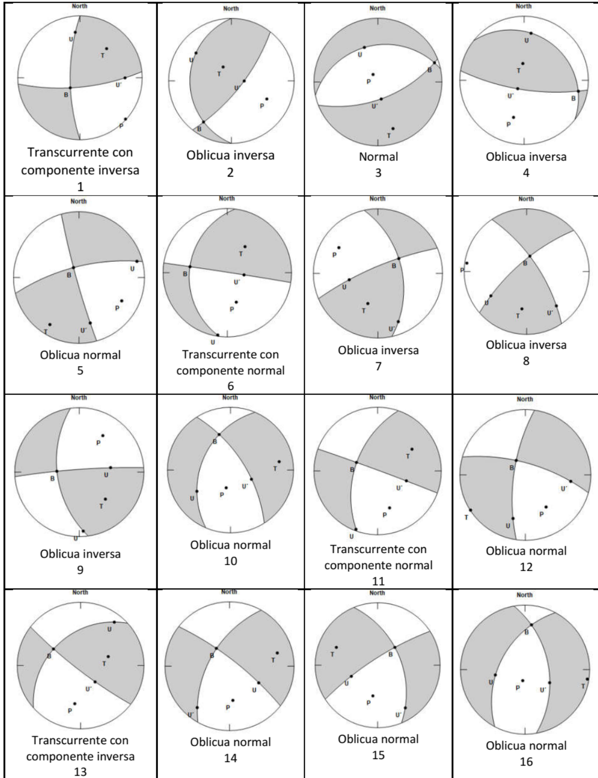
Figura 13: Gráficos de los balones de playa para los 32 sismos seleccionados. La numeración corresponde al orden de la tabla 1, en la parte inferior se especifica el tipo de falla asociada al diagrama. (Fuente: Autores.)
