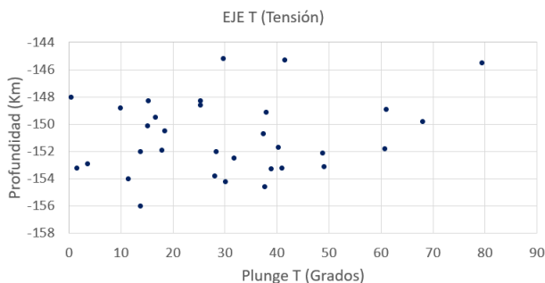
Figura 12: Representación de los ángulos de inmersión (Plunge) del eje de esfuerzos T. (Fuente: Autores.)
