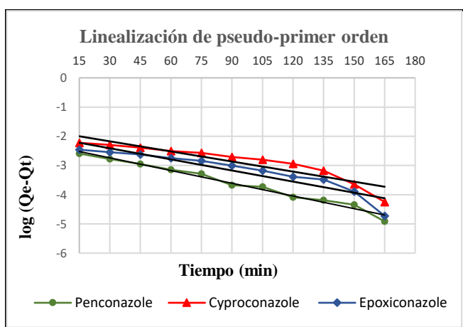
Figura 2.- Modelización de la cinética de adsorción. Pseudo-primer orden.
