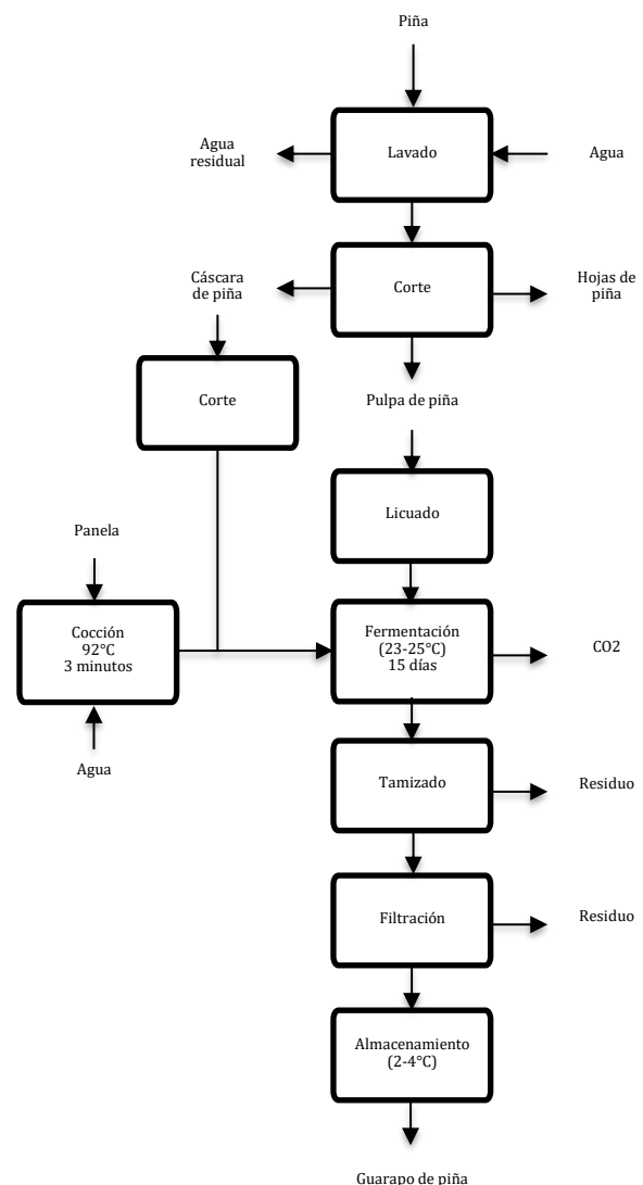
Figura 2. Diagrama de flujo de la elaboración del guarapo con fermentación controlada.
