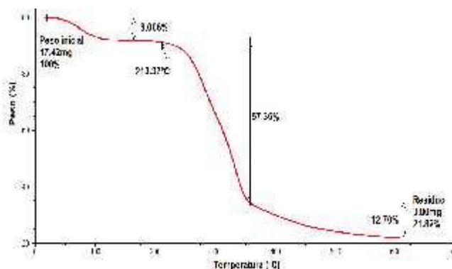
Figura 4. Termograma TG de la fibra de esparto.
