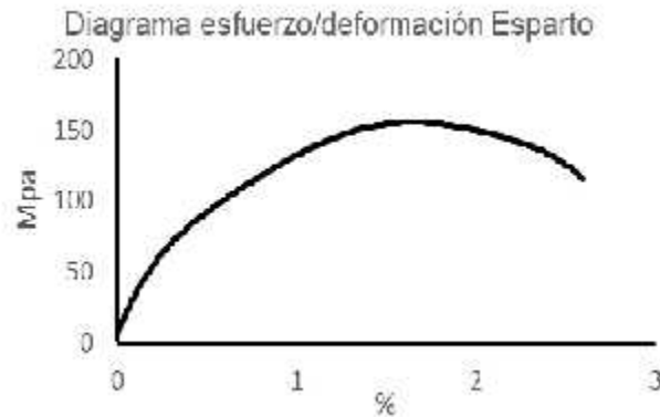
Figura 2. Diagrama esfuerzo deformación de la fibra de esparto.
