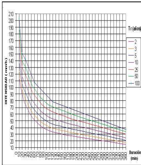
Figura 7. Curva IDF- Estación Santa Isabel
